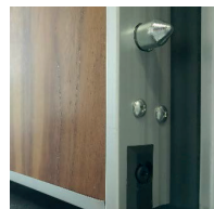
Carenado inferior , con cortavientos desmontable y 4 bulones antipalanca , en el lado de las bisagras.
